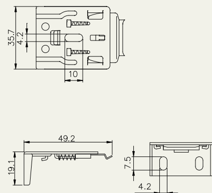
ブラケット寸法図
