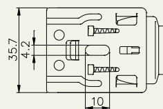
ブラケット寸法図
